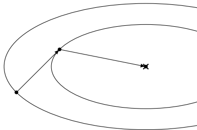
Рис.: Сопряжённые градиенты.
