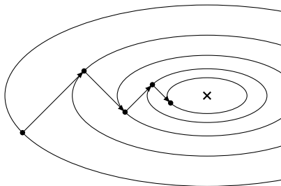
Рис.: Наискорейший спуск.
